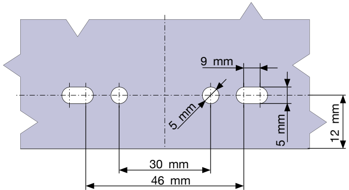
HALTEWINKEL RÜCKSEITE BACK MOUNTING BRACKET
